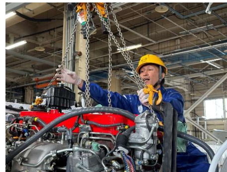
介エンジンマウントの位置出しを慎重に行う齋藤メカと福田メカ介
